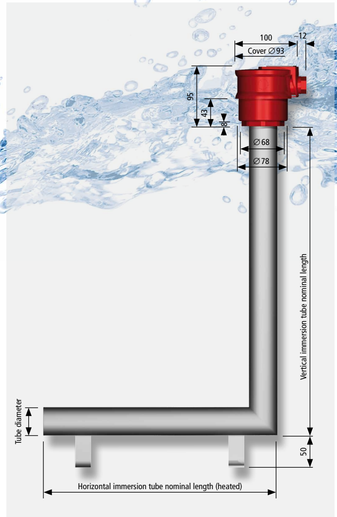
ROTKAPPE Angular Immersion Heater
